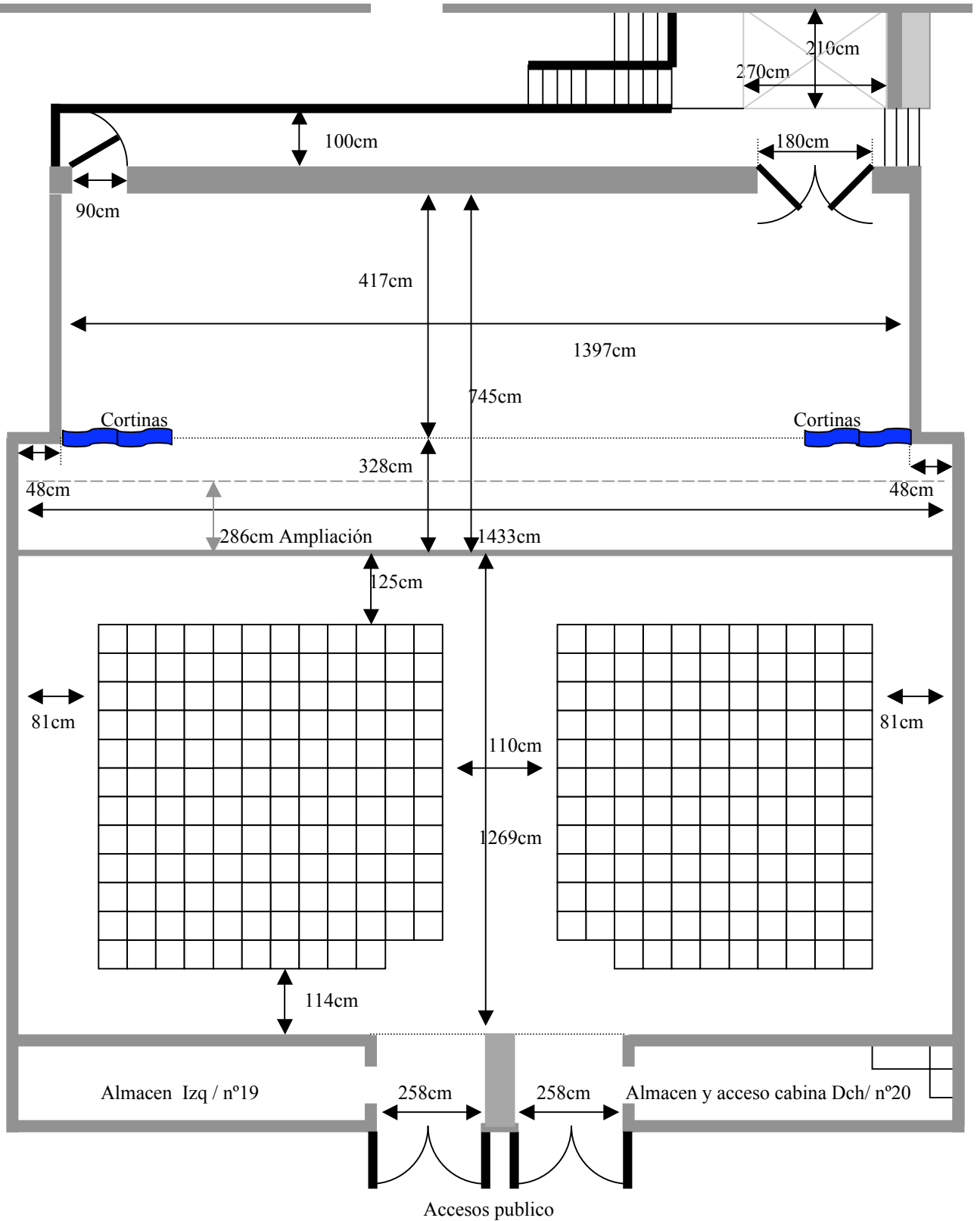
Auditorio de Galicia Croquis de la planta Sala Mozart
